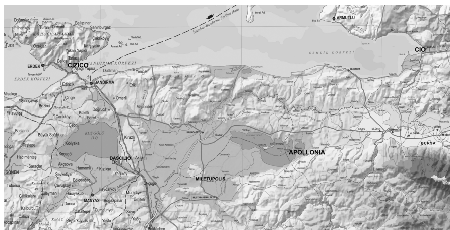
Fig. 1: Costa sud-est del Mare di Marmara.
